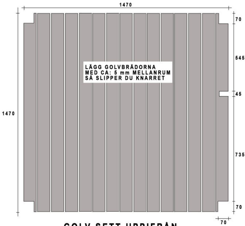
GOLV SETT UPPIFRÅN
