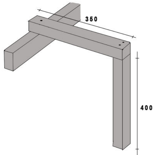
KONSOL TILL SITTBÄNK BYGG 3 ST LIKADANA
